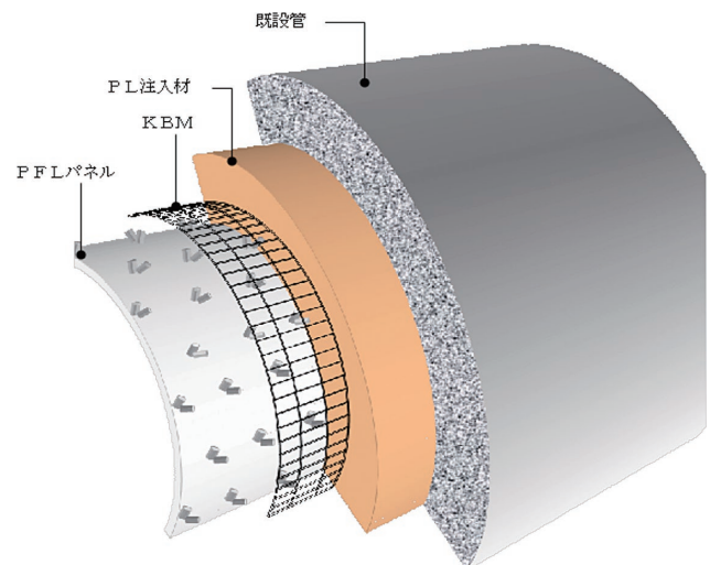
図-1 PFL工法の概要図
